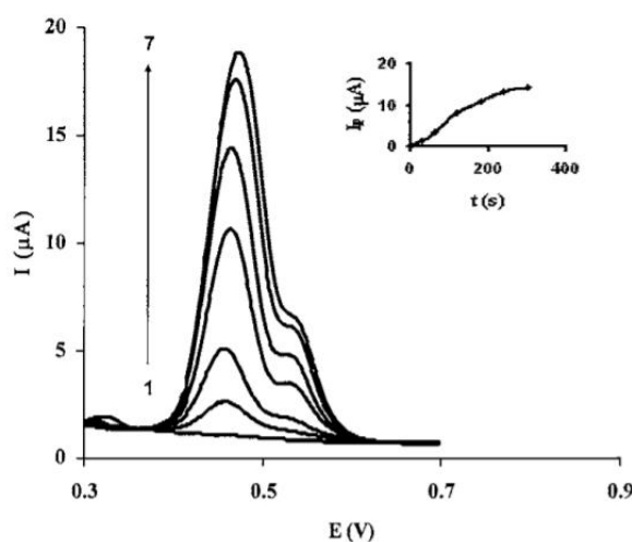
Slika 24. Diferencijalno pulsni voltamogrami 4 \mu\text{M} otopine klopapina pri različitim vremenima akumulacije (od 0 do 300 s) [40]
