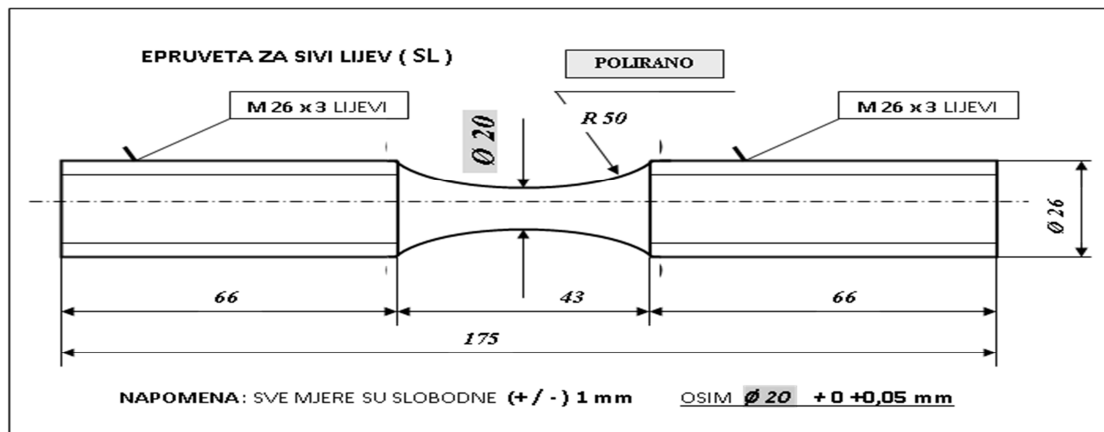
Slika 58. Izgled epruvete za statičko vlačno ispitivanje [23]
