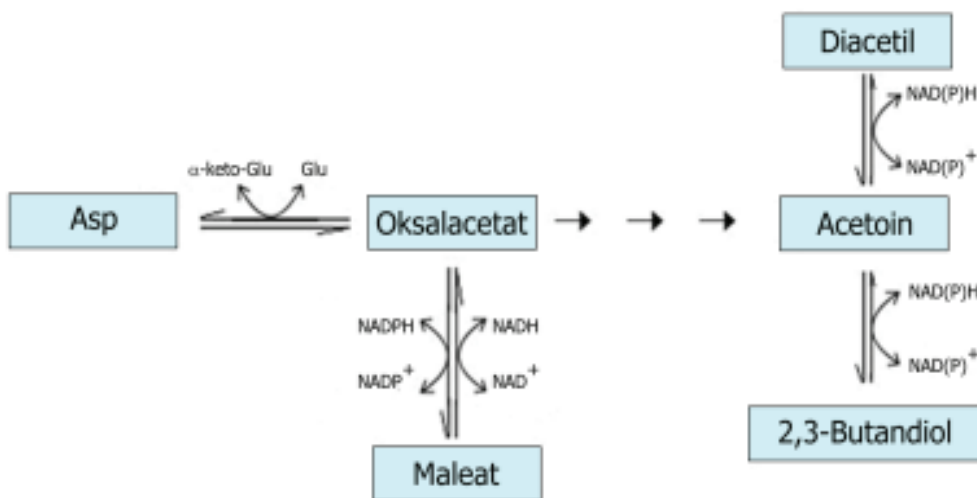
Slika 9. Shema puteva razgradnje asparaganske kiseline tijekom zrenja sira 18
