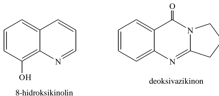
Slika 13. Alkaloidi u ekstraktima meda kestena
