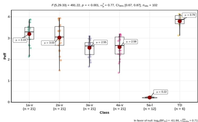
Slika 23. Usporedba permeabilnosti S+Peff ( \text{cm/s} \times 10^4 ) serije trans - \beta -laktamskih urea 1a-v i 2a-v i hidantoina 3a-v i 4a-v , parazoantina 5a-l i amida TD . S+Peff (ezetimib) = 5,34 \times 10^4 \text{ cm s}^{-1}
