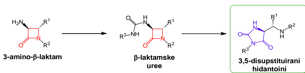
Shema 1. Općeniti sintetski put priprave kiralnih 3,5-disupstituiranih hidantoina i derivata parazoantina
