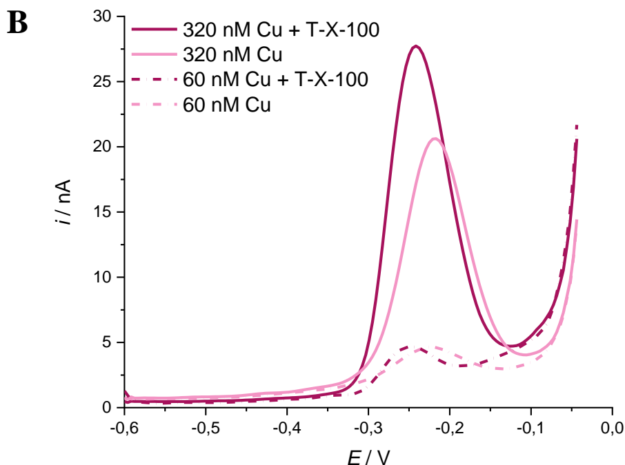
Slika 16. A) Titracijska krivulja bakra u uzorku potpovršinske vode (12_JULW) sa i bez dodatka površinski aktivne tvari, [T-X-100] = 1 mg/L, vrijeme dušiciranja 300 s, E_a = -0,6 V, t_a = 120 s, E_d = -1,4 V, B) DPASV voltamogrami bakra za [Cu^{2+}] = 60 i 320 nM, bez i sa dodatkom 1 mg/L T-X-100.
