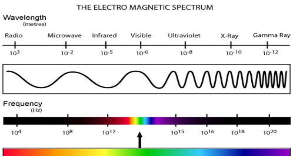
Slika 1. Elektromagnetski spektar 10
