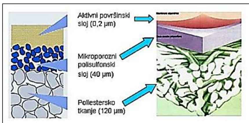
Slika 13. Sastav membrane. 20
