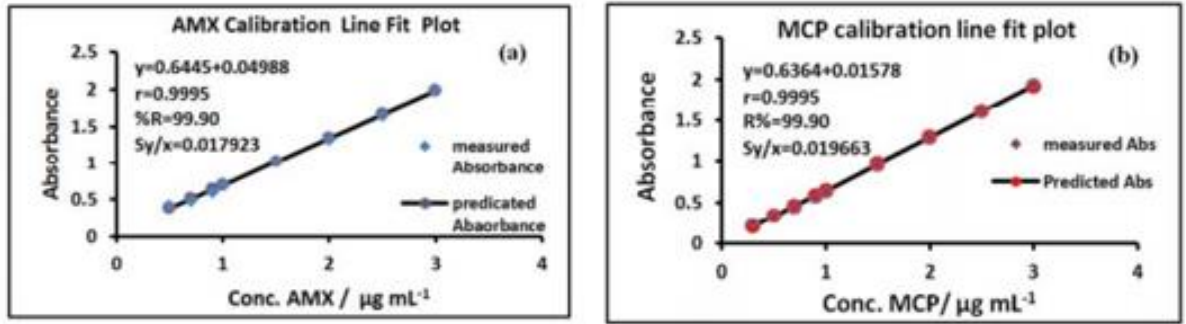
Slika 21: Kalibracijske krivulje za (a) AMX; (b) MCP 35
