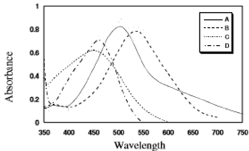
Slika 15: Apсорpcijski spektar reakcije između diazonijevе soli i (A) senidazolom, (B) niklozamidom, (C) nifuroksazidom i (D) sulfasalazinom. 27
