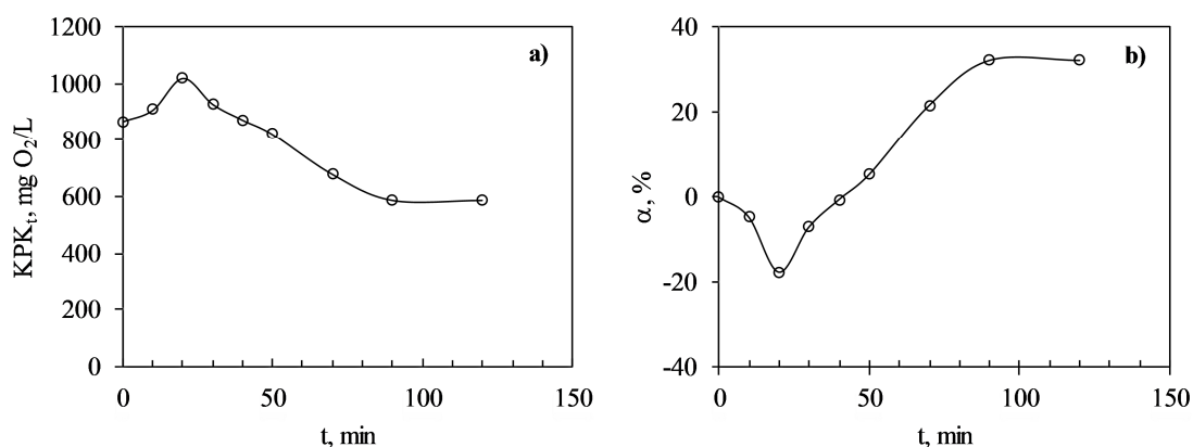
Slika 4.12. Utjecaj vremena kontakta na: (a) promjenu KPK i (b) učinkovitost smanjenja KPK .
