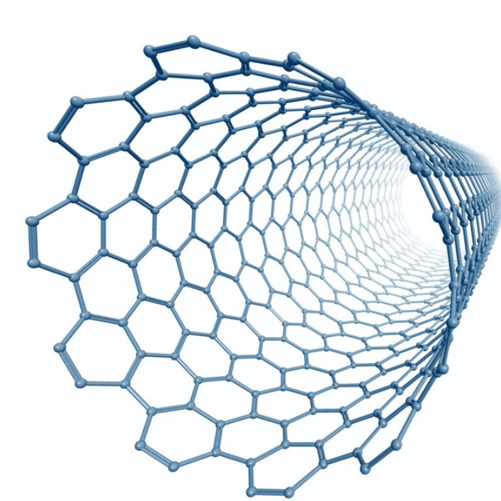
Slika 10. Struktura SWCNT [20]
