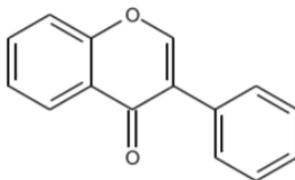
Slika 10. Struktura izoflavona. [10]
