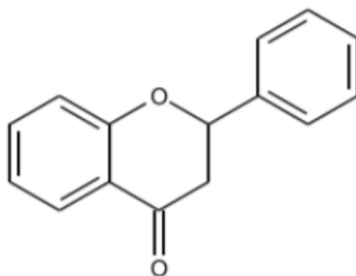
Slika 8. Struktura flavanona. [10]
