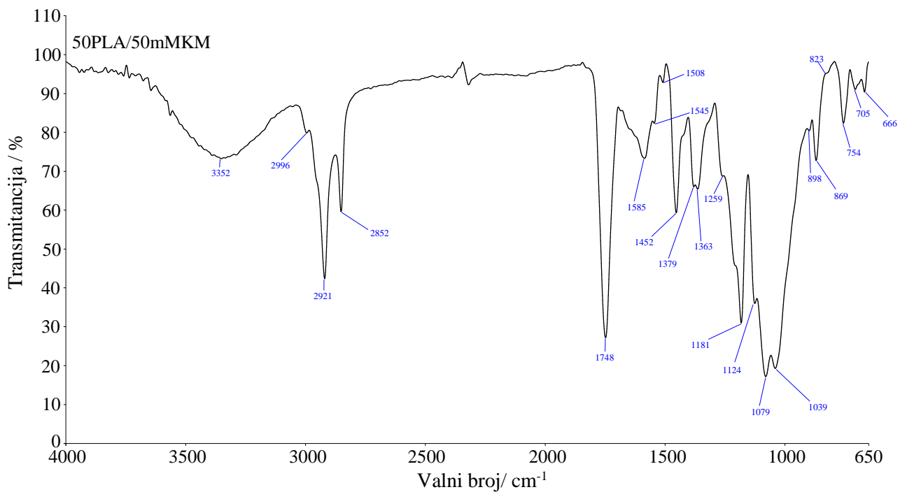
Slika 25. FT-IR spektar kompozita 50PLA/50mMKM
