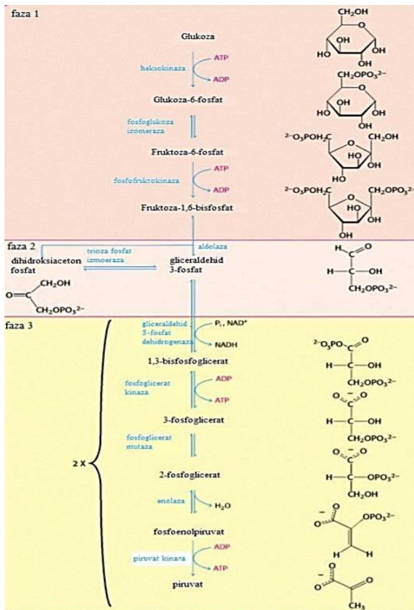
Slika 4: Glikoliza [12]
