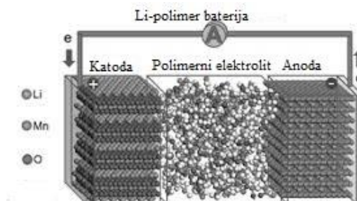
Slika 9. Li-polimer baterije 23
