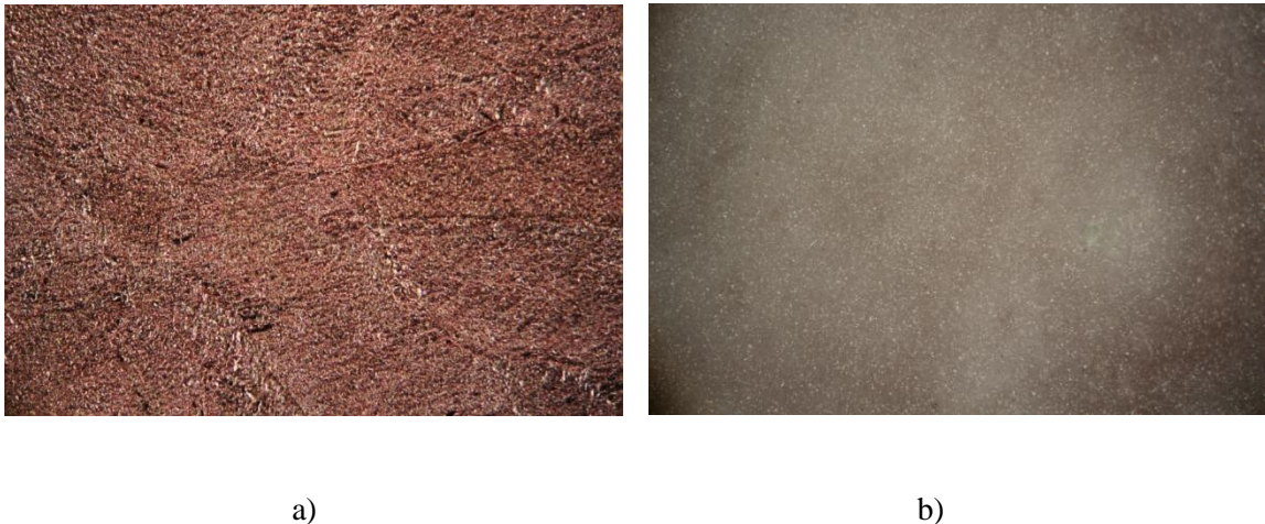
Slika 26. Snimke površine CuAlMn elektrode (uvećanje 200 puta) nakon potenciodinamičke polarizacije u 0.5 \text{ mol dm}^{-3} \text{ NaCl} + 0.3 \text{ mol dm}^{-3} \text{ Na}_2\text{SO}_4 otopini a) bez uklanjanja površinskog sloja korozivskih produkata; b) uz ultrazvučno uklanjanje površinskih produkata u deioniziranoj vodi
