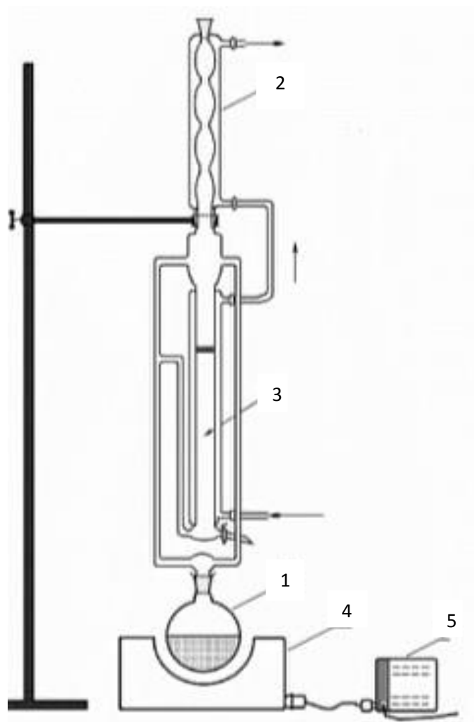
Slika 9. Shematizacija modificirane aparature prema Clevenger-u. 8
