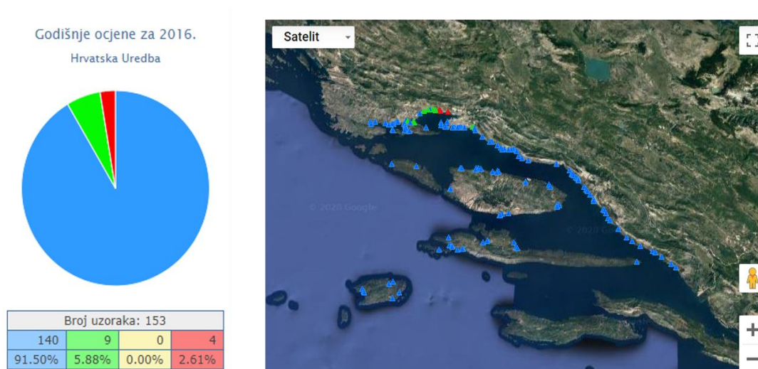
Slika 2.5. Kakvoća mora po postajama na području Splita i županije 2016. 28
