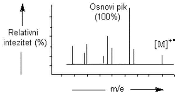
Slika 10. Spektar masa. 4
