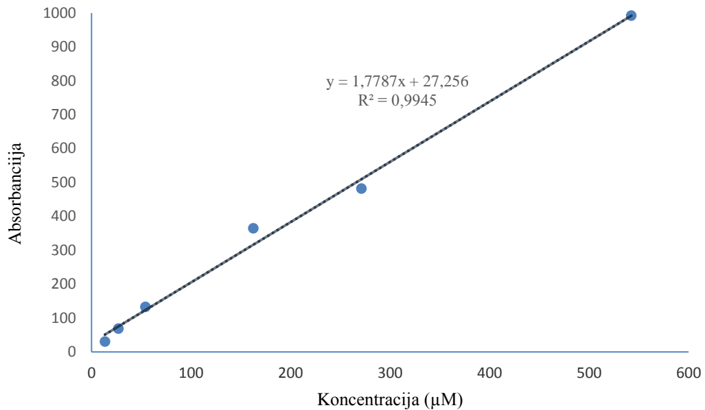
Slika 41. Baždarna krivulja sinigrina.
