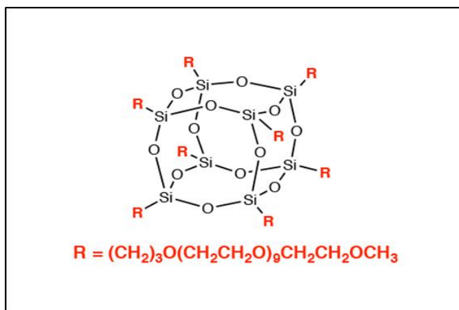
Slika 6. Struktura PEG-a 12
