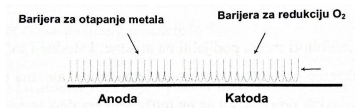
Slika 8. Adsorpcijski inhibitori.
