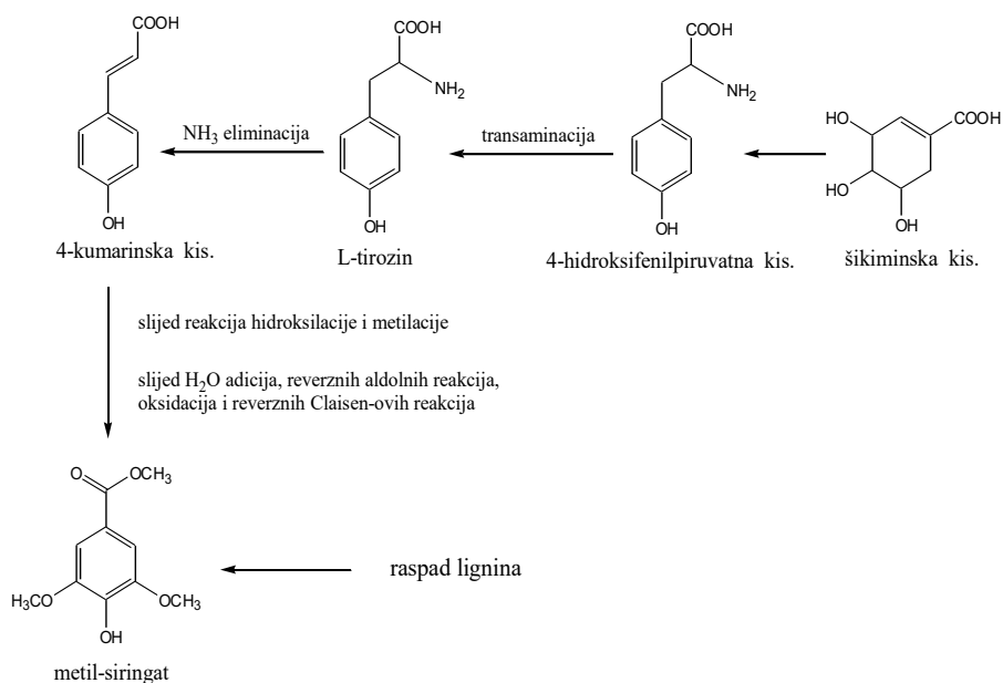
Slika 16. Biosinteza metil-siringata (43)
