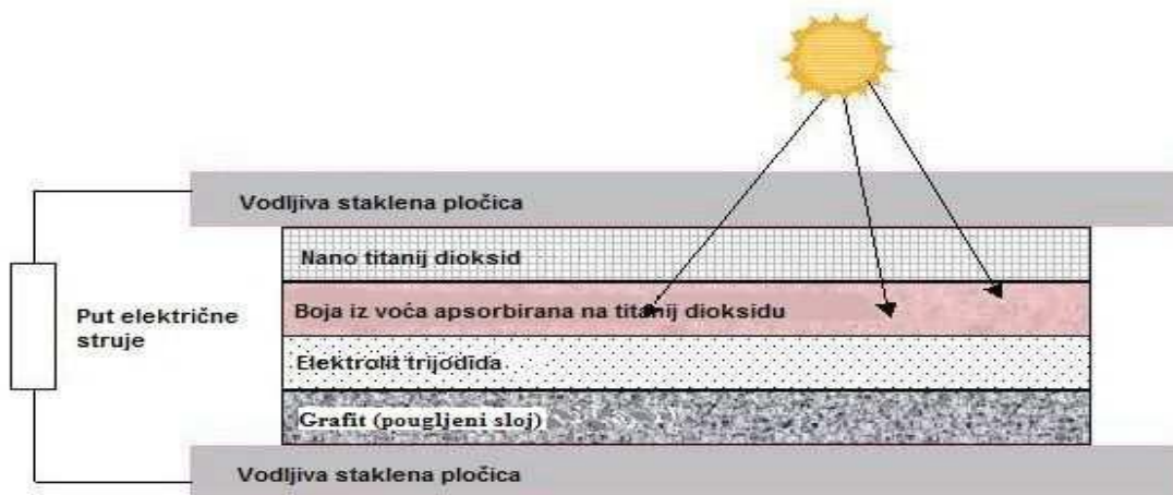
Slika 12. Shematski prikaz Grätzelove solarne ćelije 18
