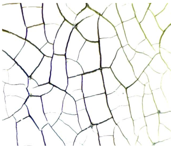
Slika 32. Izgled nanokristaličnog TiO 2 filma uz povećanje 200X
