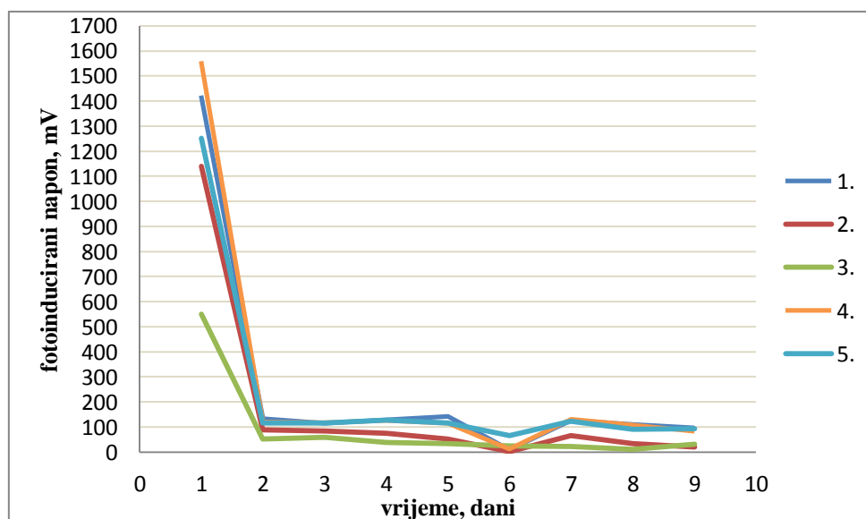
Slika 35. Ovisnost fotoinduciranog napona o vremenu pri umjetnom osvjetljenju za solarne ćelija sa slojem nanokristaličnog ZnO
