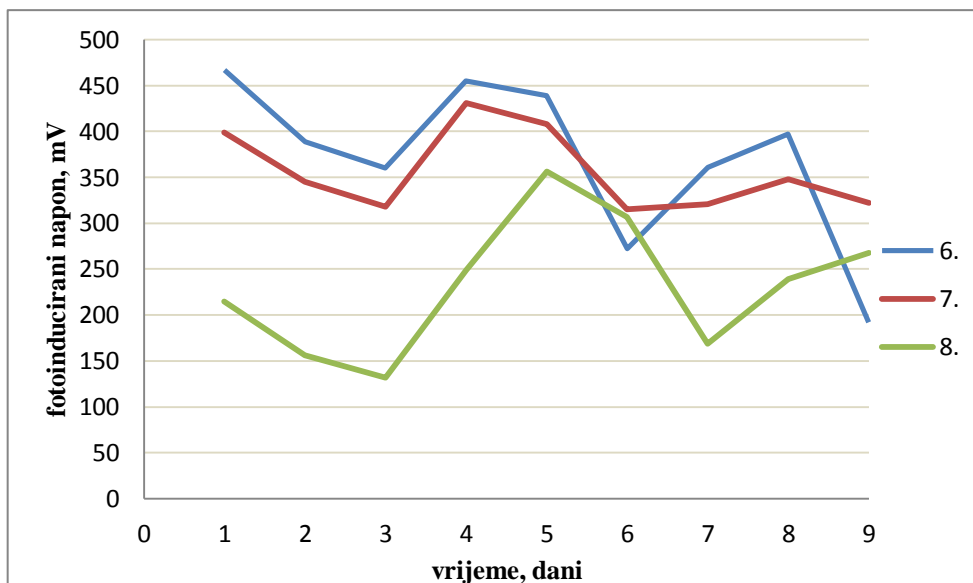
Slika 36. Ovisnost fotoinduciranog napona o vremenu pri umjetnom osvjetljenju za solarne ćelija sa slojem nanokristaličnog \text{TiO}_2
