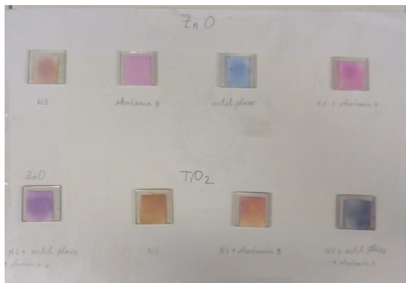
Slika 26. Osušena stakalca s oksidnim slojem i nanesenim bojilom
