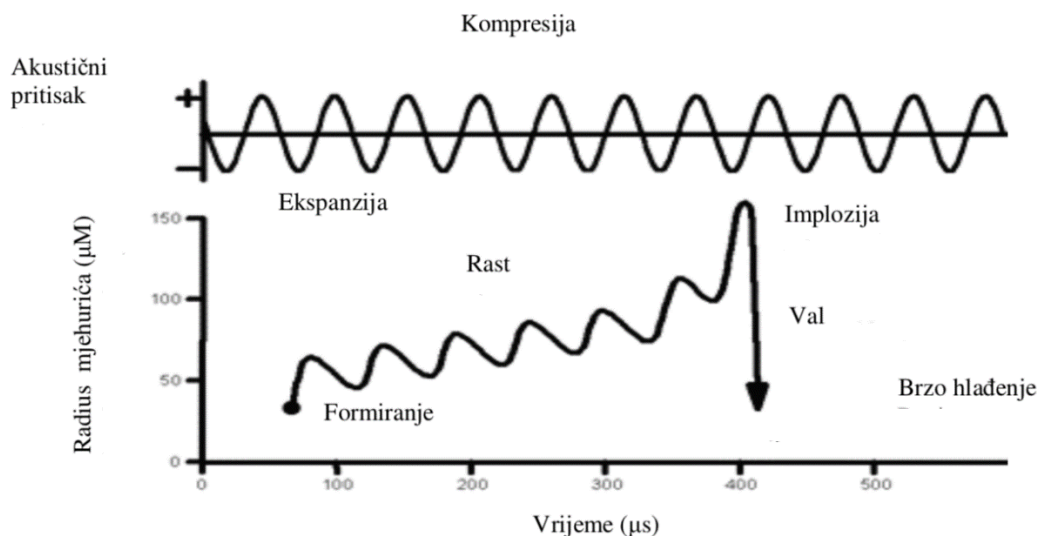
Slika 4. Djelovanje kavitacije (23)
