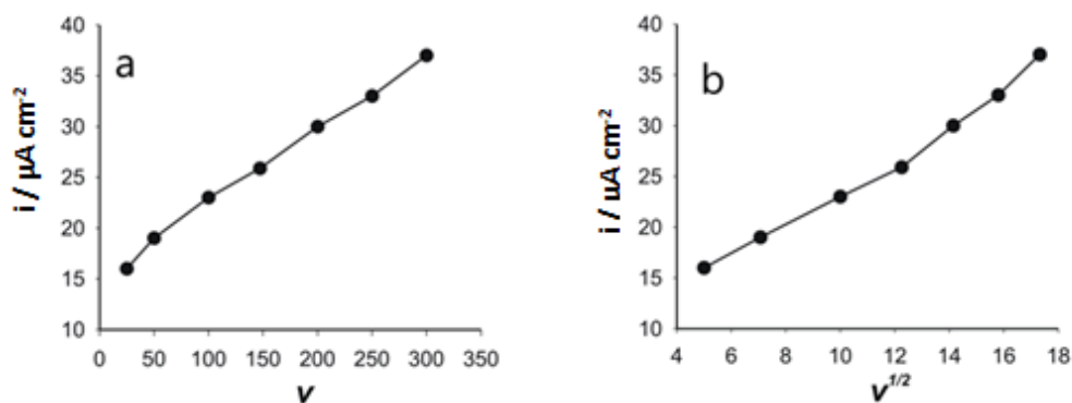
Slika 26. Utjecaj posmika na CV elektrode MWCNT-MnO 2 -30 u prisutnosti 1 \cdot 10^{-3} M H 2 O 2 pri pH 9
