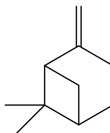
Slika 9. \beta -pinen
