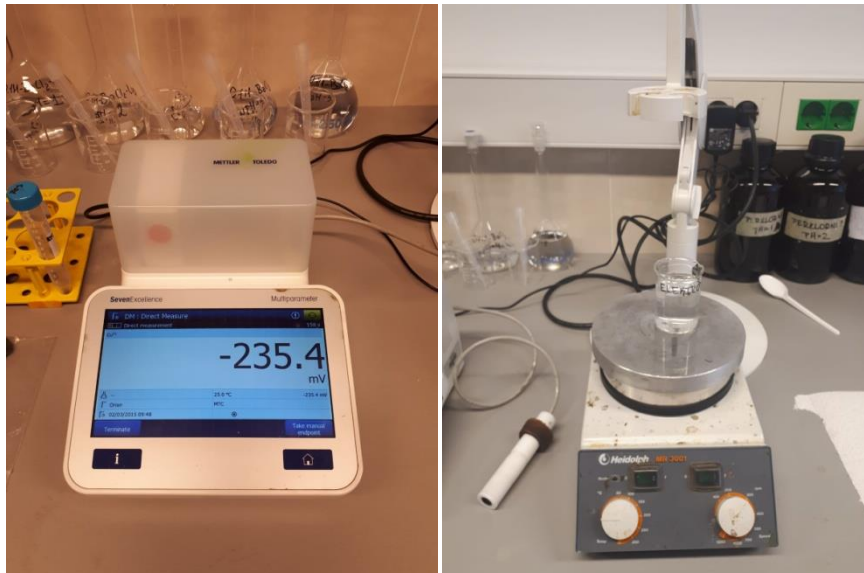
Slika 12. Potenciometrijsko mjerenje
