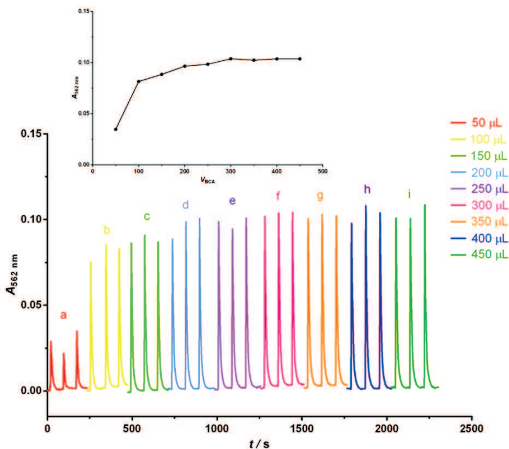
Slika 3-7 Siagram i grafički prikaz utjecaja volumena injektiranja otopine reagensa na apsorbanciju. Eksperimentalni uvjeti: osnovna otopina je deionizirana voda; otopina analita: c(\text{NACET}) = 4,0 \times 10^{-5} \text{ mol L}^{-1} ; otopina reagensa: c(\text{Cu}^{2+}) = 8,0 \times 10^{-4} \text{ mol L}^{-1} , c(\text{BCA}) = 8,0 \times 10^{-4} \text{ mol L}^{-1} , c(\text{tartarat}) = 1,6 \times 10^{-3} \text{ mol L}^{-1} ; pH = 6,8; t = 25 \text{ }^\circ\text{C} ; brzina protoka: 3000 \mu\text{L min}^{-1} ; volumen petlje zadržavanja: 1000 \mu\text{L} ; volumen reakcijske petlje: 120 \mu\text{L} ; volumen injektiranja otopine reagensa: (a) 50 \mu\text{L} , (b) 100 \mu\text{L} , (c) 150 \mu\text{L} , (d) 200 \mu\text{L} , (e) 250 \mu\text{L} , (f) 300 \mu\text{L} , (g) 350 \mu\text{L} , (h) 400 \mu\text{L} , (i) 450 \mu\text{L} ; volumen injektiranja otopine analita (NACET): 200 \mu\text{L} ; volumen osnovne otopine: 3500 \mu\text{L} ; volumen protočne kivete: 80 \mu\text{L} ; \lambda = 562 \text{ nm} .
