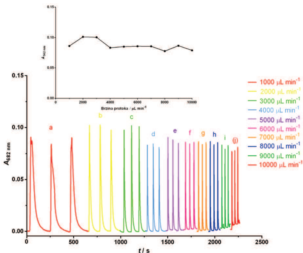
Slika 3-5 Siagram i grafički prikaz utjecaja brzine protoka na zabiljezeni signal. Eksperimentalni uvjeti: osnovna otopina je deionizirana voda; otopina analita: c(\text{NACET}) = 4,0 \times 10^{-5} \text{ mol L}^{-1} ; otopina reagensa: c(\text{Cu}^{2+}) = 8,0 \times 10^{-4} \text{ mol L}^{-1} , c(\text{BCA}) = 8,0 \times 10^{-4} \text{ mol L}^{-1} , c(\text{tartarat}) = 1,6 \times 10^{-3} \text{ mol L}^{-1} ; pH = 6,8; t = 25 \text{ }^\circ\text{C} ; brzina protoka: (a) 1000 \mu\text{L min}^{-1} , (b) 2000 \mu\text{L min}^{-1} , (c) 3000 \mu\text{L min}^{-1} , (d) 4000 \mu\text{L min}^{-1} , (e) 5000 \mu\text{L min}^{-1} , (f) 6000 \mu\text{L min}^{-1} , (g) 7000 \mu\text{L min}^{-1} , (h) 8000 \mu\text{L min}^{-1} , (i) 9000 \mu\text{L min}^{-1} , (j) 10\ 000 \mu\text{L min}^{-1} ; volumen petlje zadržavanja: 1000 \mu\text{L} ; volumen reakcijske petlje: 280 \mu\text{L} ; volumen injektiranja otopine reagensa: 200 \mu\text{L} ; volumen injektiranja otopine analita (NACET): 200 \mu\text{L} ; volumen osnovne otopine: 3500 \mu\text{L} ; volumen protočne kivete: 80 \mu\text{L} ; \lambda = 562 \text{ nm} .
