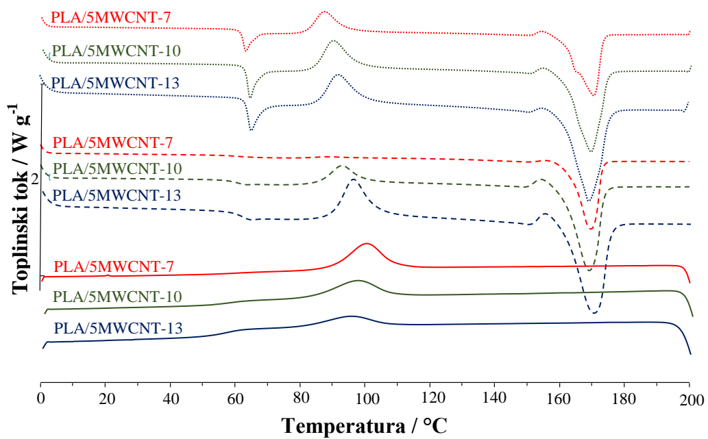
Slika 25. DSC krivulje prvog zagrijavanja, hlađenja i drugog zagrijavanja PLA/5MWCNT kompozita snimljene pri brzinama zagrijavanja/hlađenja 7, 10 i 13 ^{\circ}\text{C min}^{-1}
