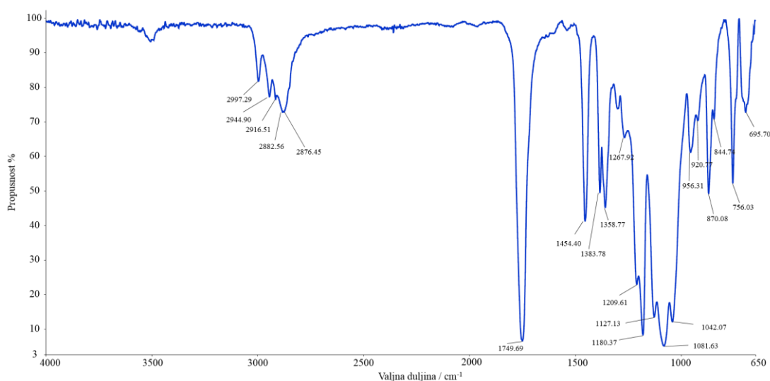
Slika 28. FTIR spektrogram mješavine PLA/PEO (80/20)
