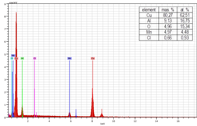
Slika 28. a) SEM snimka CuAlMn legure nakon potenciodinamičkog polarizacijskog mjerenja u 0,9% NaCl otopini ( pH = 7,4 ) pri T = 24^\circ C s označenim točkom za EDS analizu; b) EDS analiza površine
