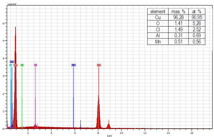
Slika 29. a) SEM snimka CuAlMn legure nakon potenciodinamičkog polarizacijskog mjerenja u 0,9% NaCl otopini ( pH = 7,4 ) pri T = 50^\circ C s označenim točkom za EDS analizu; b) EDS analiza površine
