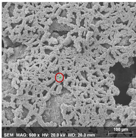
Slika 29. a) SEM snimka CuAlMn legure nakon potenciodinamičkog polarizacijskog mjerenja u 0,9% NaCl otopini ( pH = 7,4 ) pri T = 50^\circ C s označenim točkom za EDS analizu; b) EDS analiza površine
