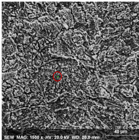
Slika 28. a) SEM snimka CuAlMn legure nakon potenciodinamičkog polarizacijskog mjerenja u 0,9% NaCl otopini ( pH = 7,4 ) pri T = 24^\circ C s označenim točkom za EDS analizu; b) EDS analiza površine
