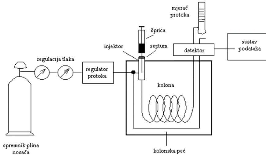
Slika 13. Shematski prikaz plinske kromatografije Izvor: http://free-zg.t-com.hr/Svjetlana_Luterotti/09/091/0912.htm
