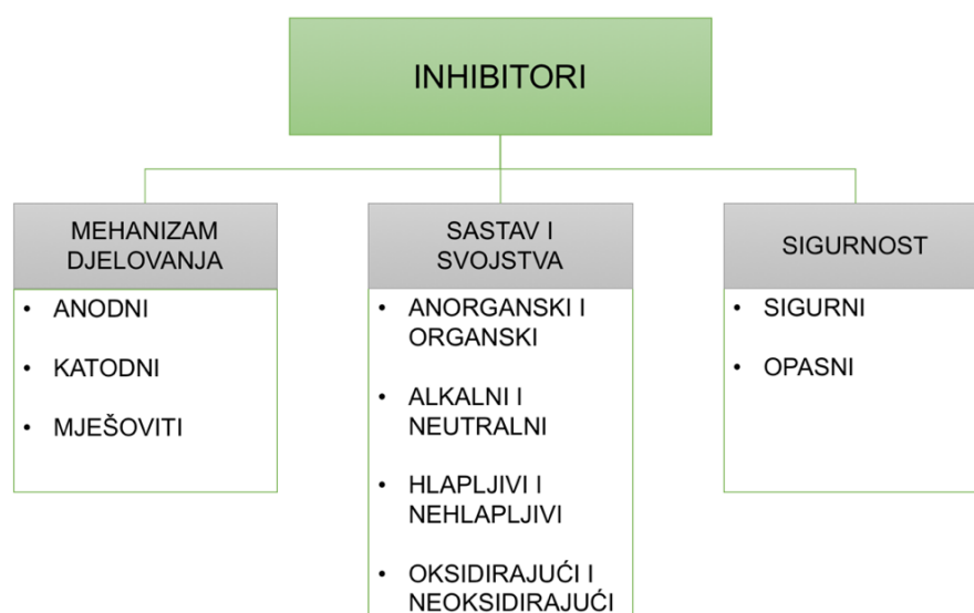
Slika 10. Klasifikacija inhibitora.
