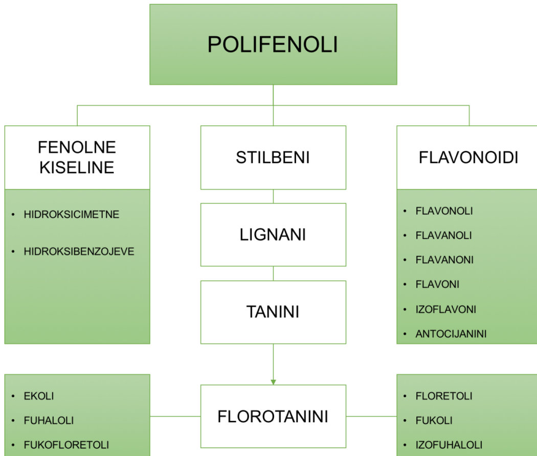
Slika 25. Klasifikacija polifenola.
