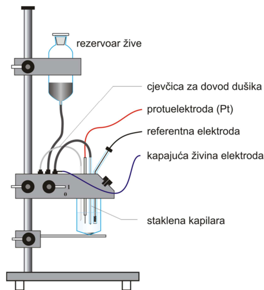
Slika 7. Shematski prikaz sustava za polarografsko mjerenje
