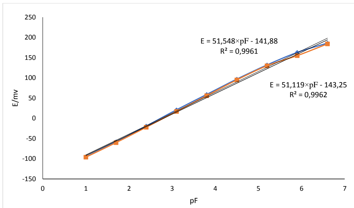
Slika 4.7. Ovisnost promjene potencijala s promjenom koncentracije F^- za FISE metodom slijednog razrjeđenja
