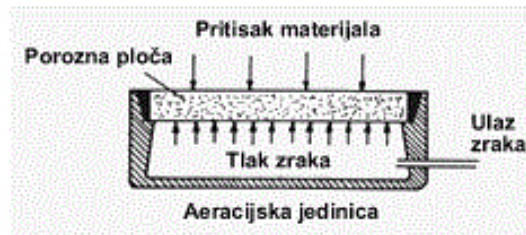
Slika 3. Aeracijska jedinica [7]
