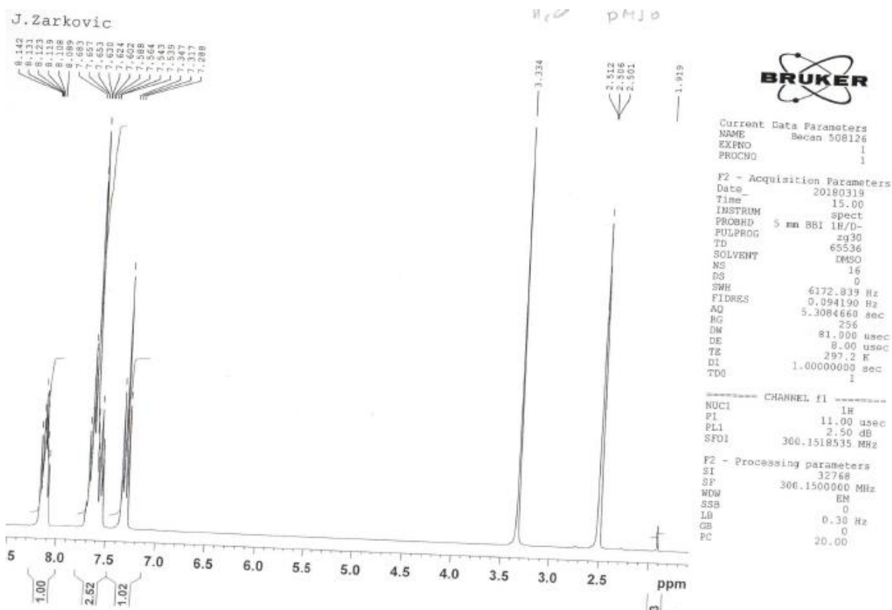
Slika 6.8. ^1\text{H} -NMR spektar spoja 5b
