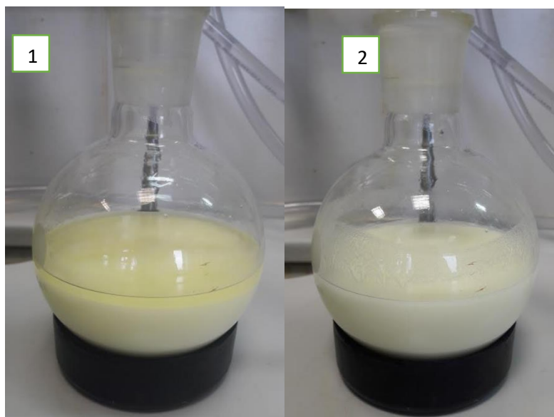
Slika 2.33. Na slici 1 je prikazana još vruća otopina tek skinuta s refluksa. Slika 2 prikazuje ohlađenu otopinu.
