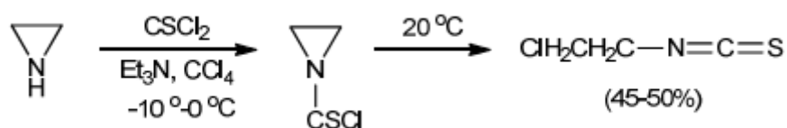
Slika 2.10. Reakcija aziridina i tiofोजना, te nastanak izotiocijanata. 8
