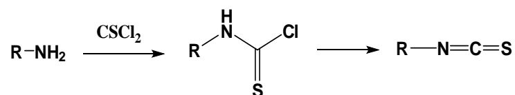
Slika 8. Sinteza izotocijanata reakcijom primarnog amina s tiofuzgenom 8
