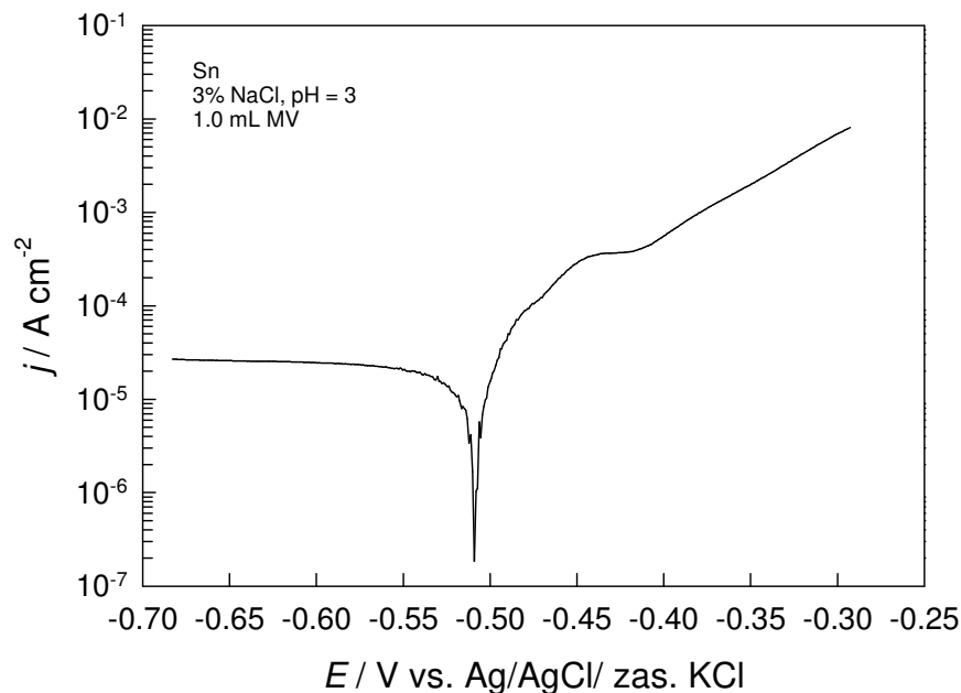
Slika 3.10. Tafelov prikaz polarizacijske krivulje elektrode od kositra u 3%-tnoj otopini NaCl, pH = 3.0 uz dodatak 1 mL MV, snimljene brzinom promjene potencijala od 10 \text{ mV s}^{-1}
