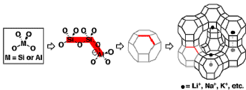
Slika 1.8. Struktura zeolita 15
