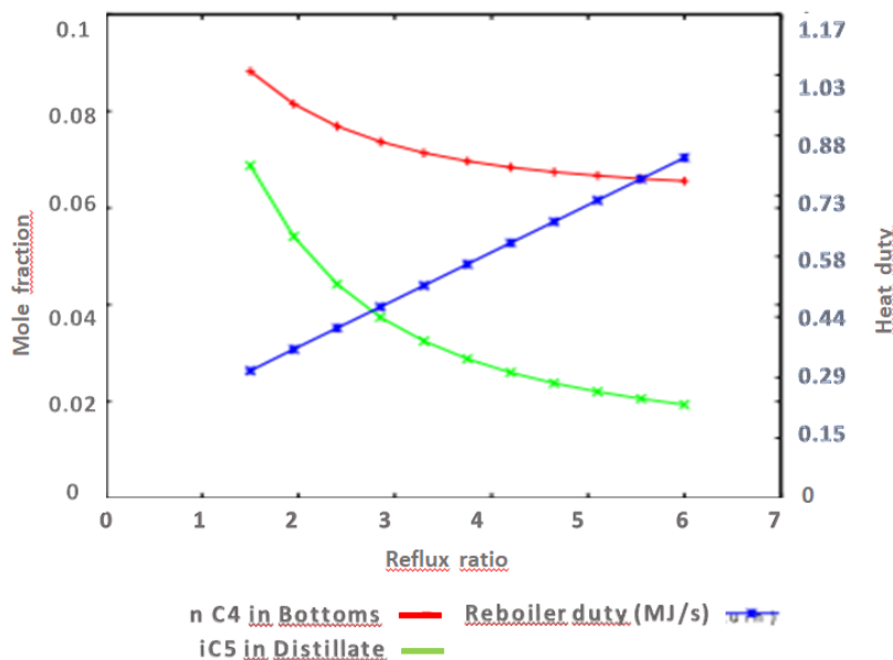
Slika 4.11. Grafički prikaz utjecaja refluksnog omjera na molni udio n-butana u proizvodu dna i izopentana u destilatu te toplinsku dužnost rebojlera.
