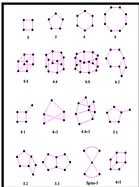
Slika 4. Sekundarne strukturne jedinice zeolita (SBU) 21
