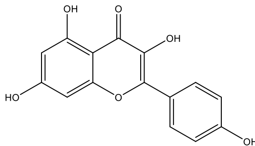
Kempferol
