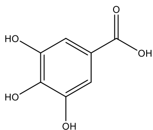
Galna kiselina
