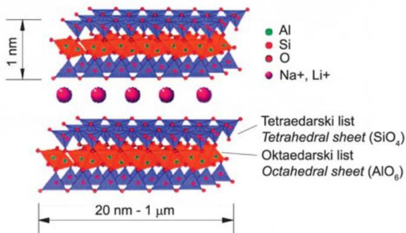
Slika 4. Struktura 2:1 filossilikata 9
